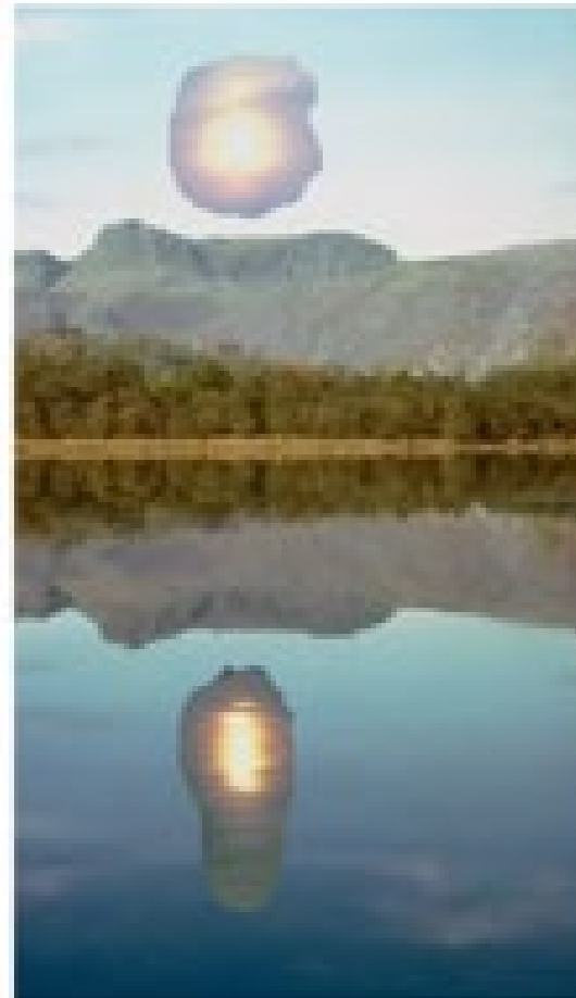
copy-paste
